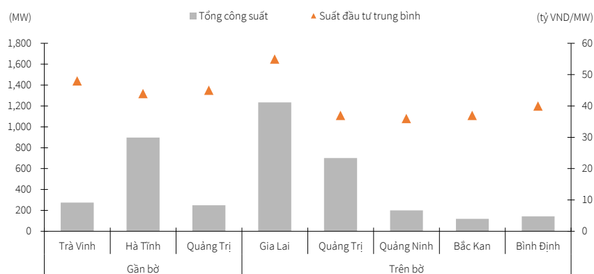
Biểu đồ 13. Phân bổ công suất và suất đầu tư điện gió mới nhất của các tỉnh
